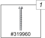
Betonschraube mit Sechskantkopf BSZ2-SU 10x90 Concrete screw with hexagon head BSZ2-SU 10x90
