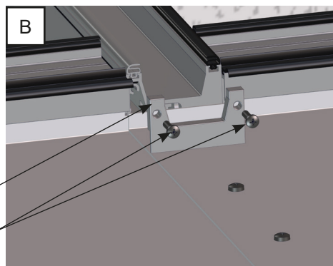
Montage der Abdeckkappen an den Modulstößen Installation of the cover caps on the module joints
