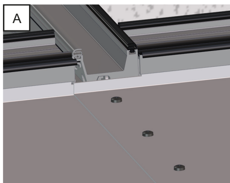
Montage der Abdeckkappen an den Modulstößen Installation of the cover caps on the module joints
