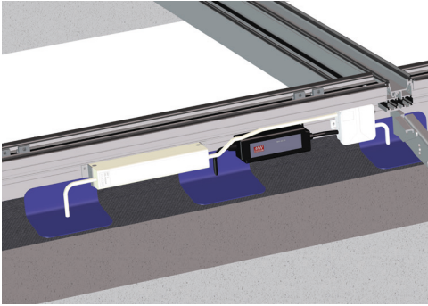
Elektrischer Anschluss für öffnenbaren Flügel mit innenliegender Verschattung Electrical connection for openable sash with internal shading
