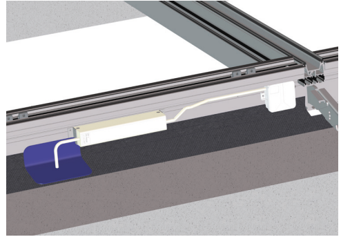
Elektrischer Anschluss für öffnenbaren Flügel ohne innenliegender Verschattung Electrical connection for openable sash without internal shading
